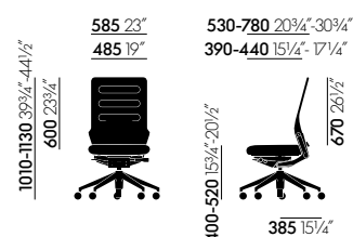
AC 5 Work ohne Armlehnen, mit verstellbarer Lumbalstütze
