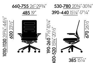
AC 5 Work mit FreeFloat-Armlehnen und verstellbarer Lumbalstütze
