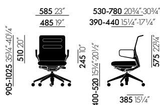
AC 5 Work Lowback mit Ringarmlehnen
