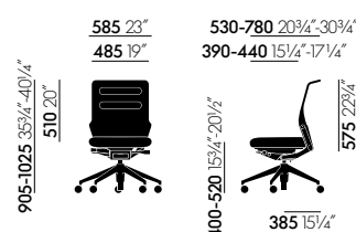
AC 5 Work Lowback ohne Armlehnen
