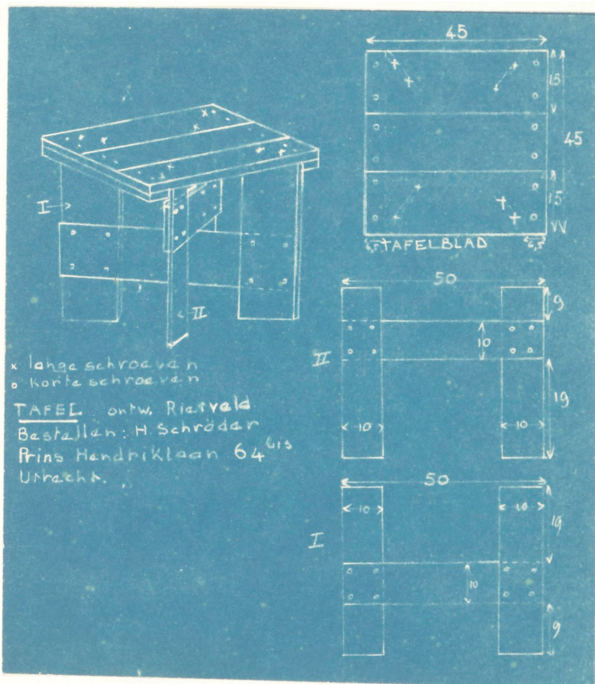
Blue print of Crate Low Table by Gerrit Rietveld, 1934. Centraal Museum Utrecht, Stichting Auteursrechten G. Th. Rietveld
